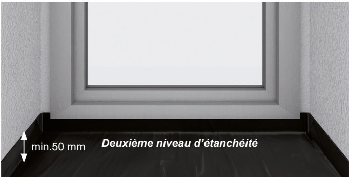
III. 4 : Représentation schématique du second niveau d'étanchéité en forme de cuvette.
