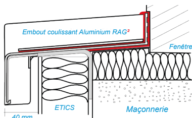
III. 2 : Représentation schématique Dimension de retrait pour RAG 2 et section transversale (toutes modifications)
